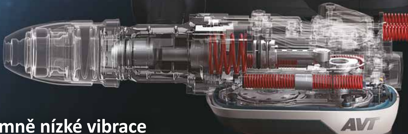
50 mm Kombinované kladivo HR5212C
